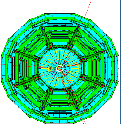
ATLAS
